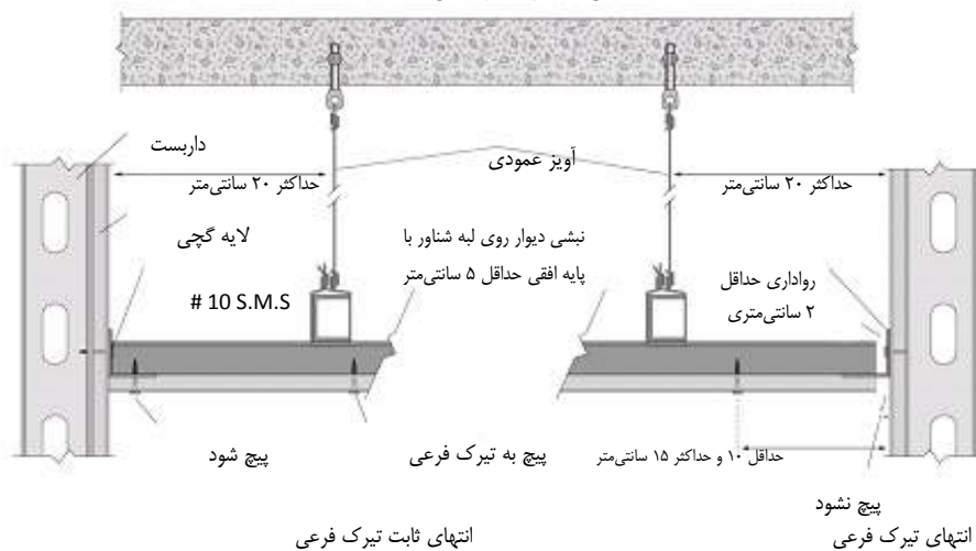
مقطع B-B: مهار تیرچه فرعی
