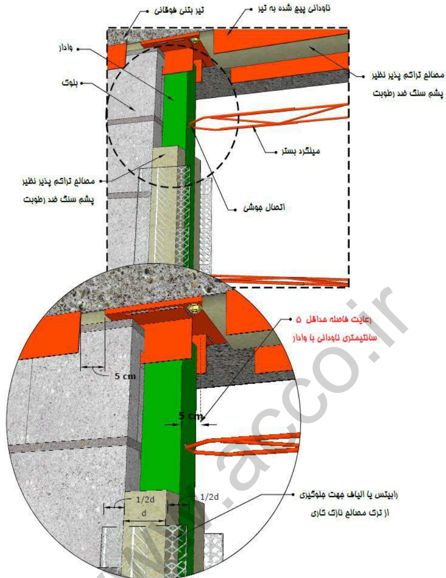
شکل پ ۴-۶-۴-۱- اتصال به وادارها
