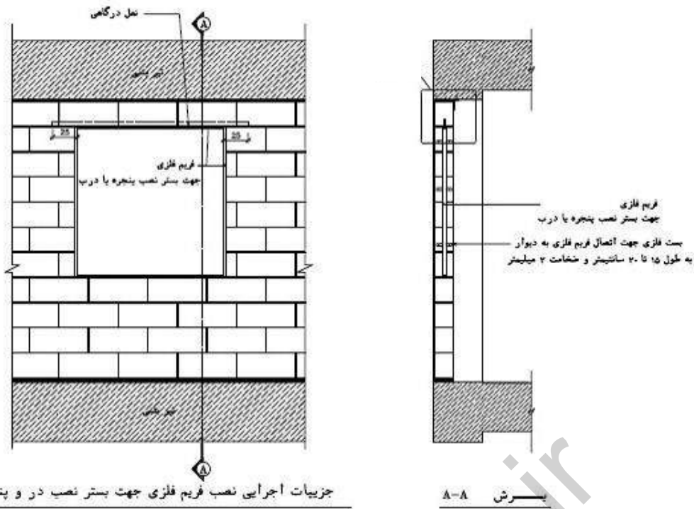
شکل پ ۶-۱۵- نحوه اجرای فریم و نعل درگاه در اطراف بازشو
